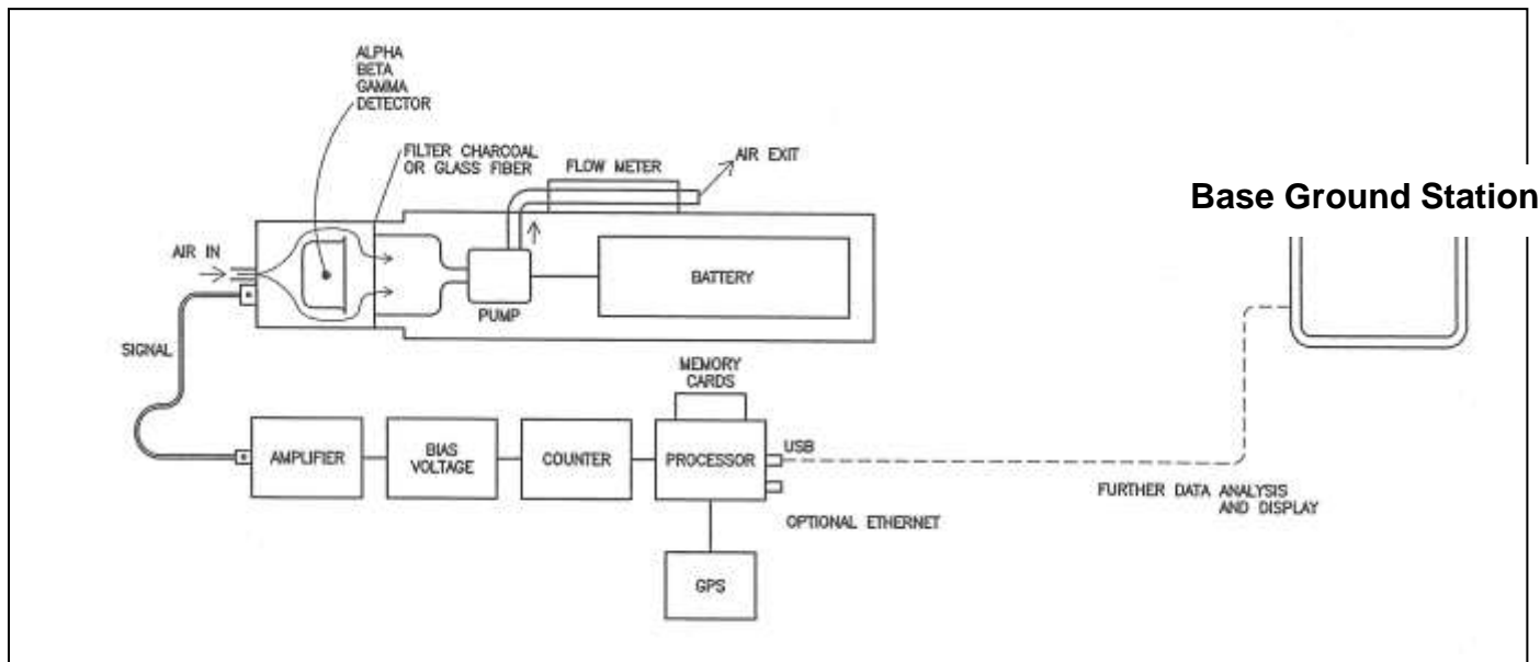
DroneRAD-P Detector Set Up
